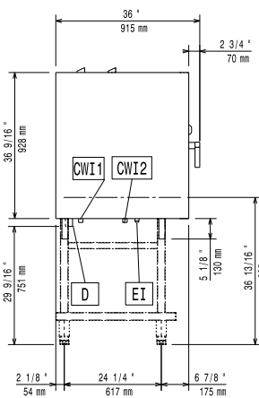
Zij aanzicht
